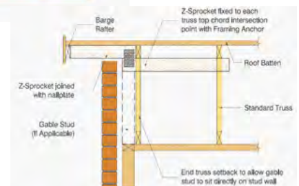
ZED SPROCKETS
